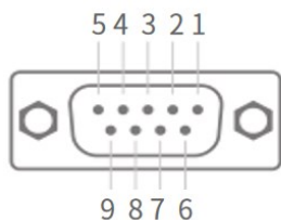
图 2-7 COM 接口示意图
