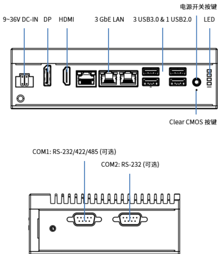
E225 接口示意图
