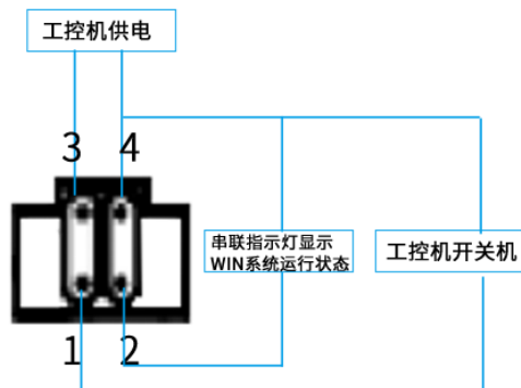
图 2-1 凤凰端子电源输入接口示意图
