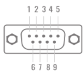
图 2-7 串口接口示意图
