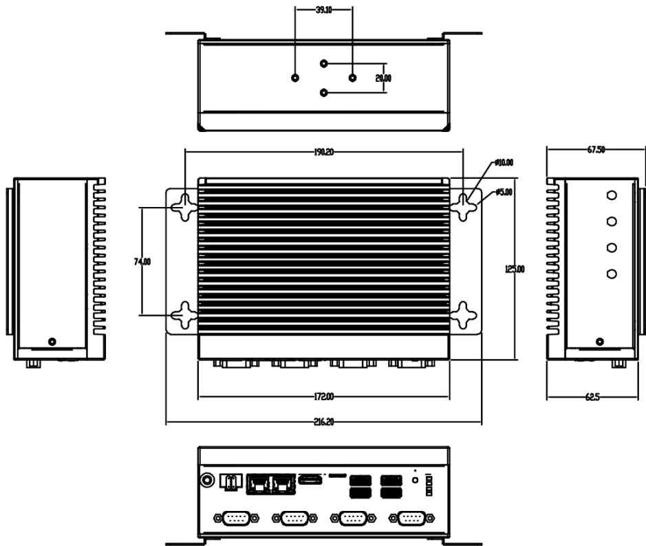
图 1-2 E200 具体尺寸图
