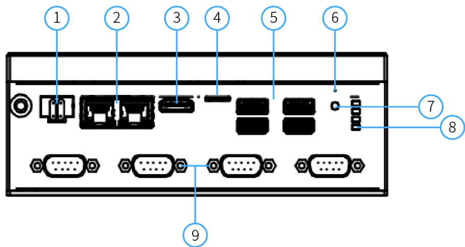
图 2-1 E200 接口说明图
